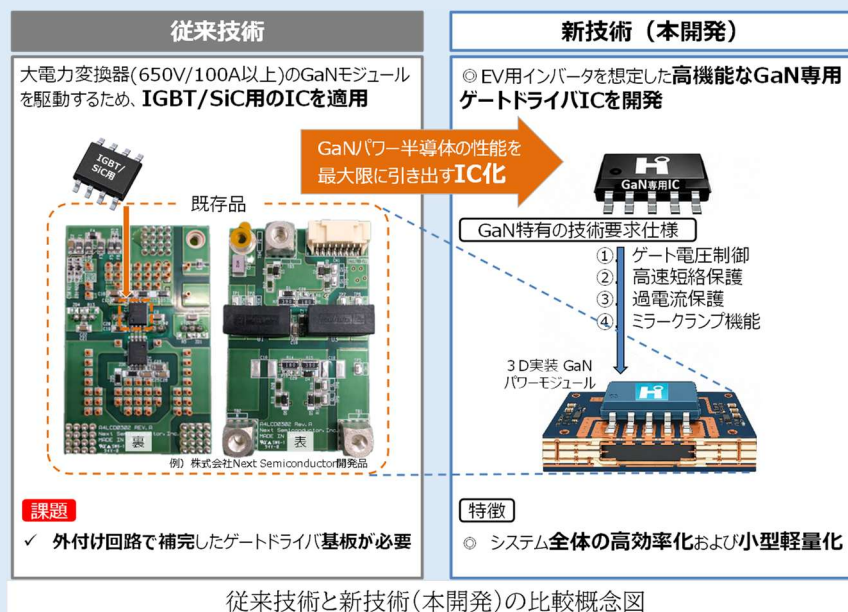
従来技術と新技術(本開発)の比較概念図
